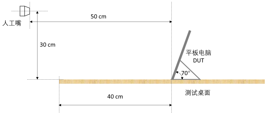
图24 平板电脑传声器测试布局图
