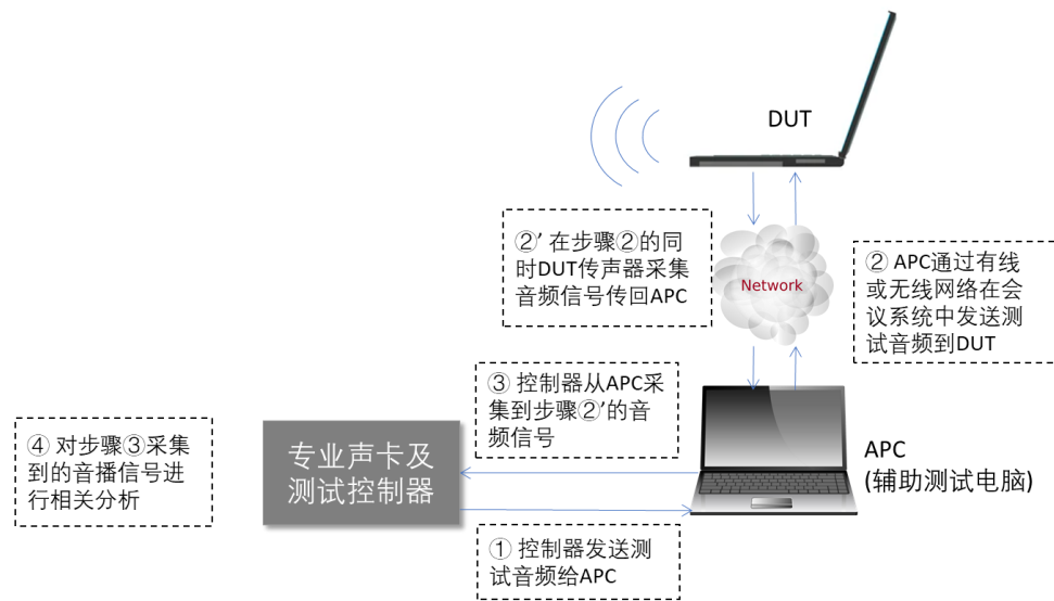
图33 DUT 回声消除幅度(单向通话)测试连接图
