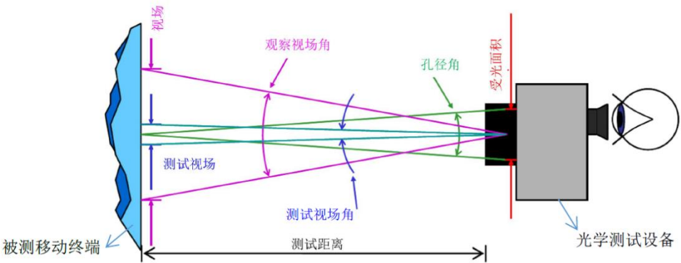
图11 显示测试设备要求
