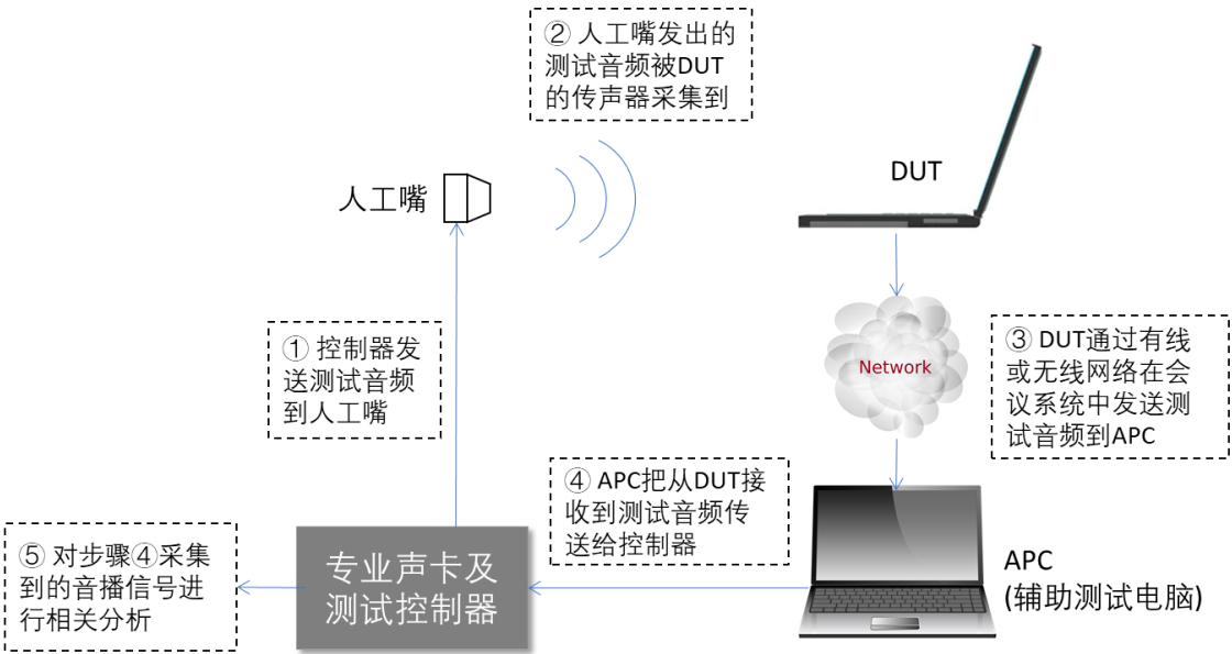
图31 DUT 传声器测试连接图
