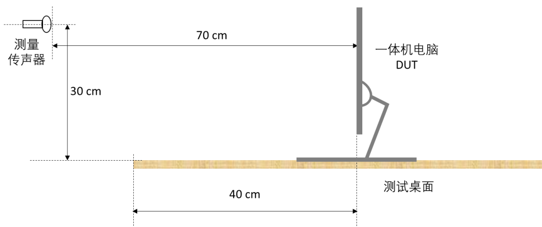
图29 一体机电脑扬声器测试布局图
