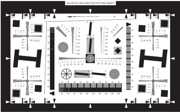
图3 可视分辨率测试图卡范例
