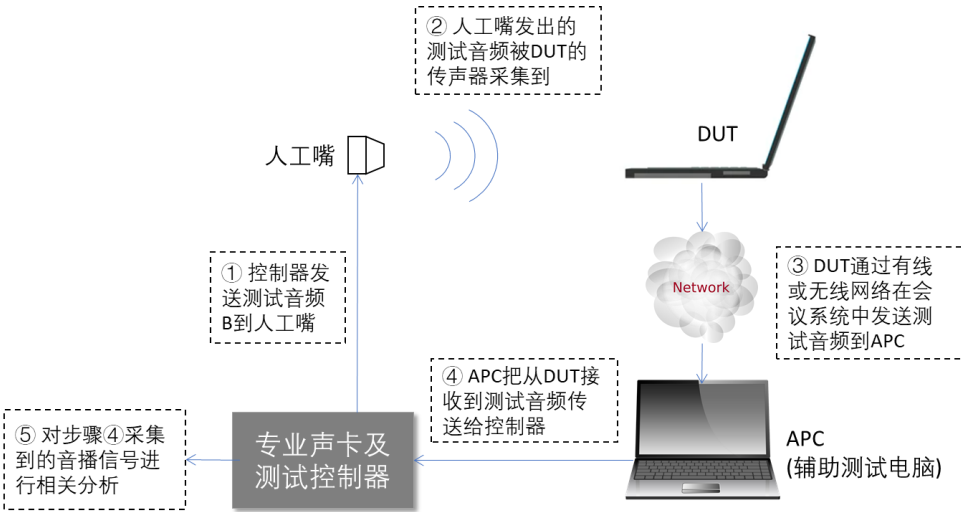
图34 回声消除幅度测试(双向同时通话)连接图 1
