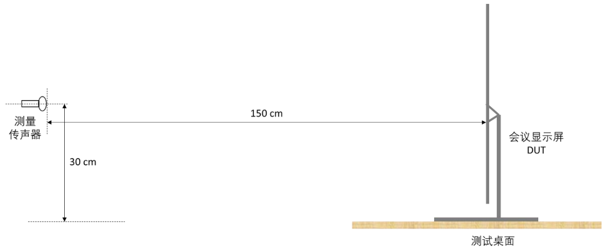
图30 会议显示屏扬声器测试布局图
