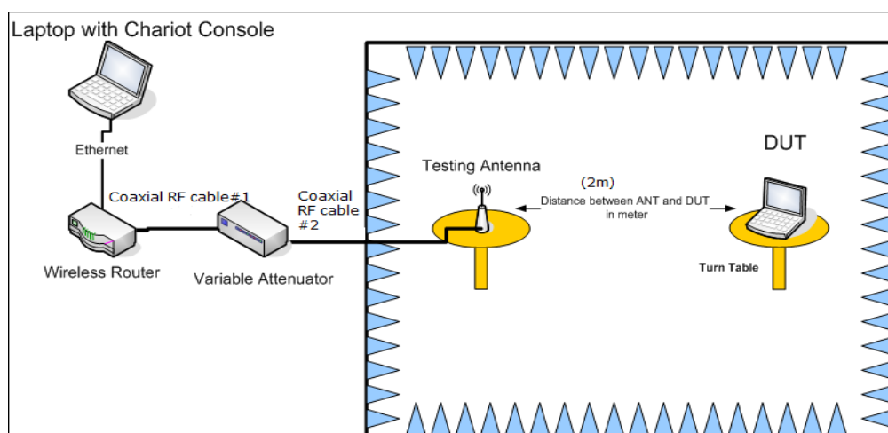
图36 吞吐量测试环境
