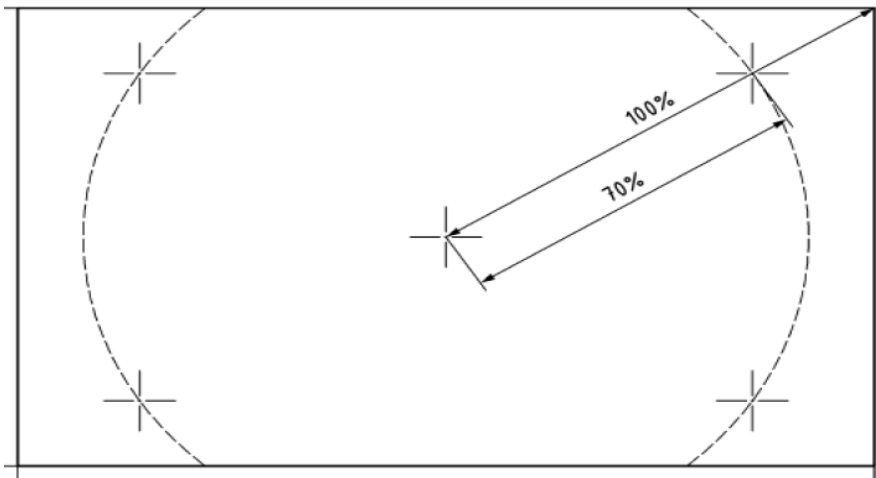
图2 可视分辨率测试中心及四角测试位置
