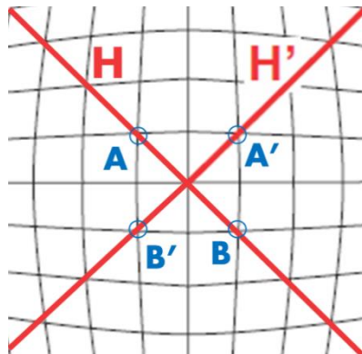
图7 畸变测试示意图
