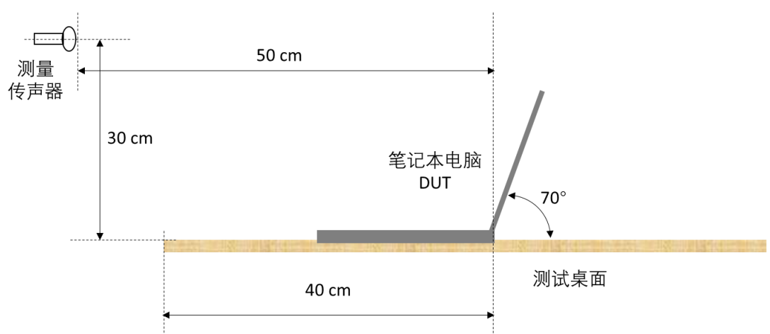
图27 笔记本电脑扬声器测试布局图
