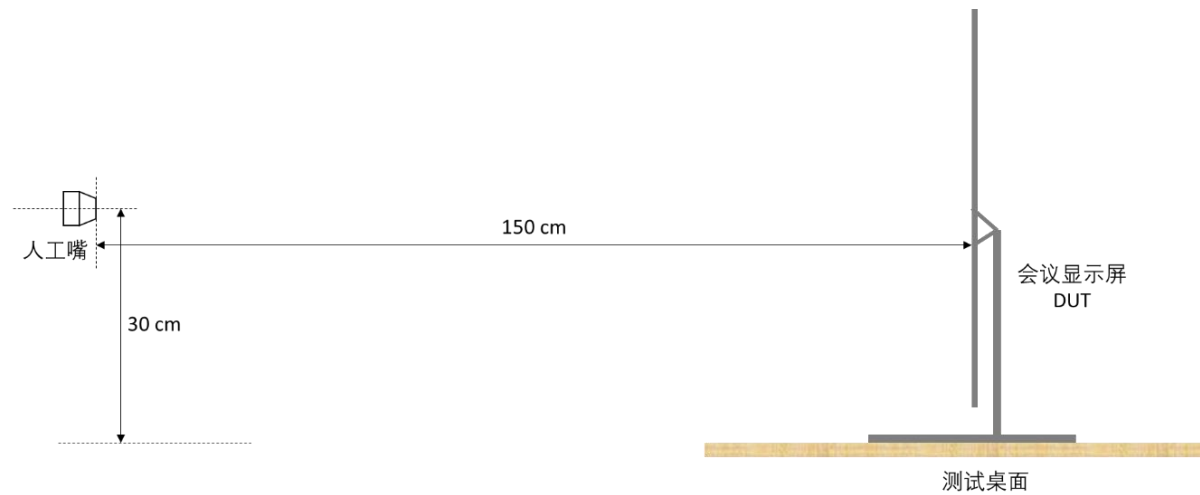
图26 会议显示屏传声器测试布局图
