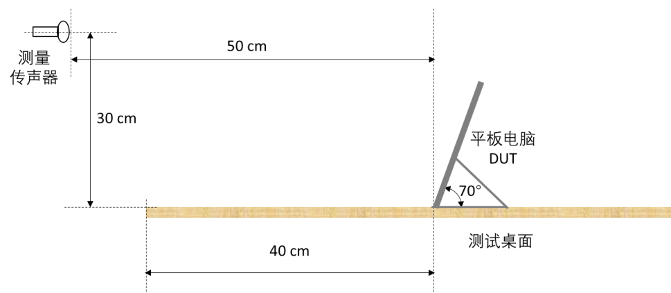
图28 平板电脑扬声器测试布局图
