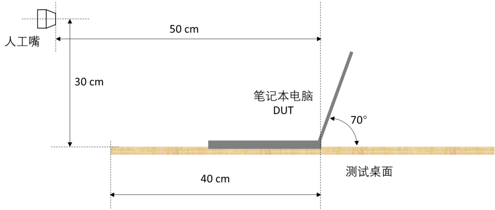
图23 笔记本电脑传声器测试布局图
