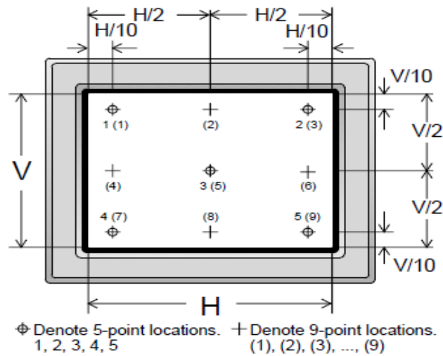
图21 九点亮度测试位置
