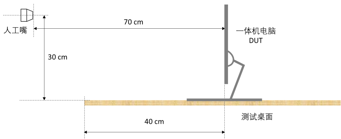
图25 一体机电脑传声器测试布局图
