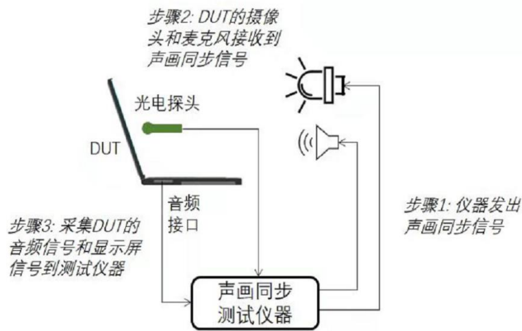
图38 音频和视频同步性测试连接图
