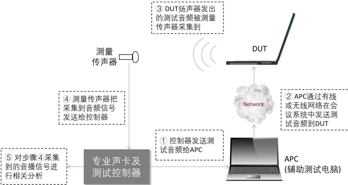
图32 DUT 扬声器测试连接图
