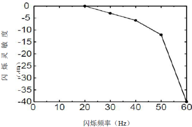
图22 人眼在不同频率下感知闪烁的灵敏度曲线
