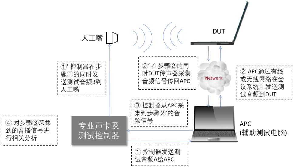
图35 回声消除幅度测试(双向同时通话)连接图 2
